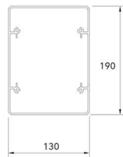
3 Профил колона
