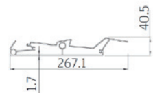
Схема при отворено положение със събрани ламели:
