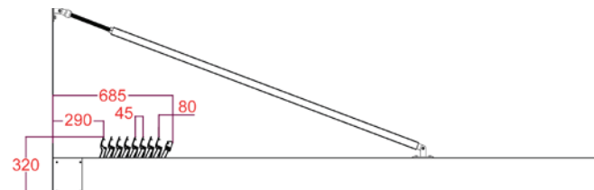
Схема при отворено положение със събрани ламели:
