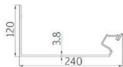
1 Заден улук
