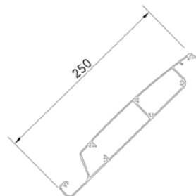
2 Ламелен профил
