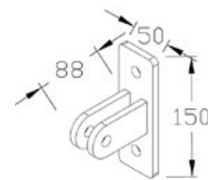
6 Предна стойка за захващане
