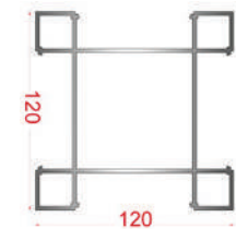
1 Профил колона
