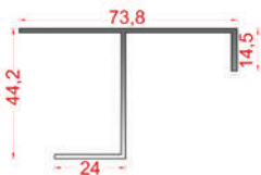
5 Заден профил
