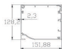
5 Кутия за мотор
