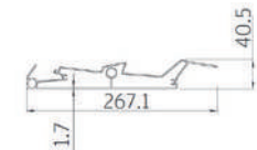
Схема при отворено положение със събрани ламели:
