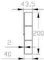
2 Преден профил
