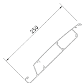
2 Ламелен профил
