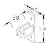
6 Предна стойка за захващане
